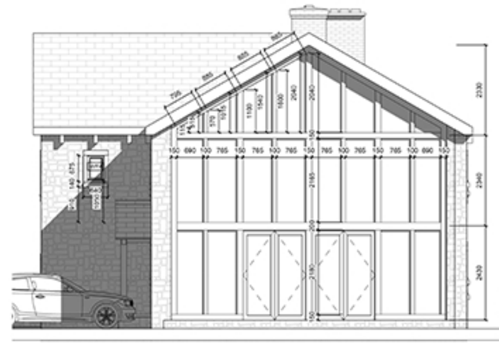
SE side elevation 1:50
